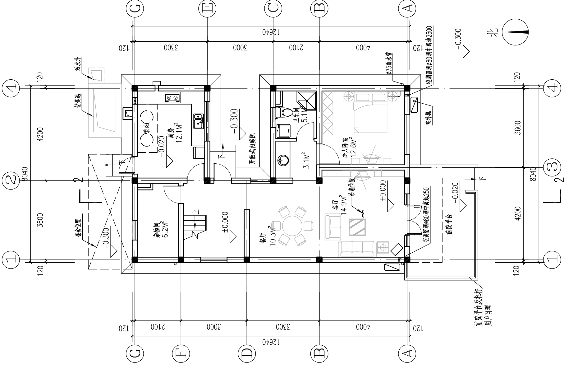
一层平面 1:100
