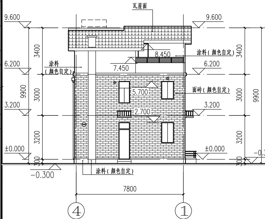
北立面图 1:150
