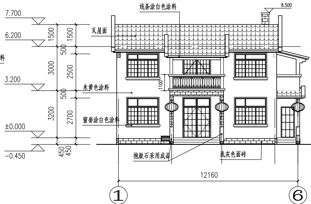
南立面 1:150
