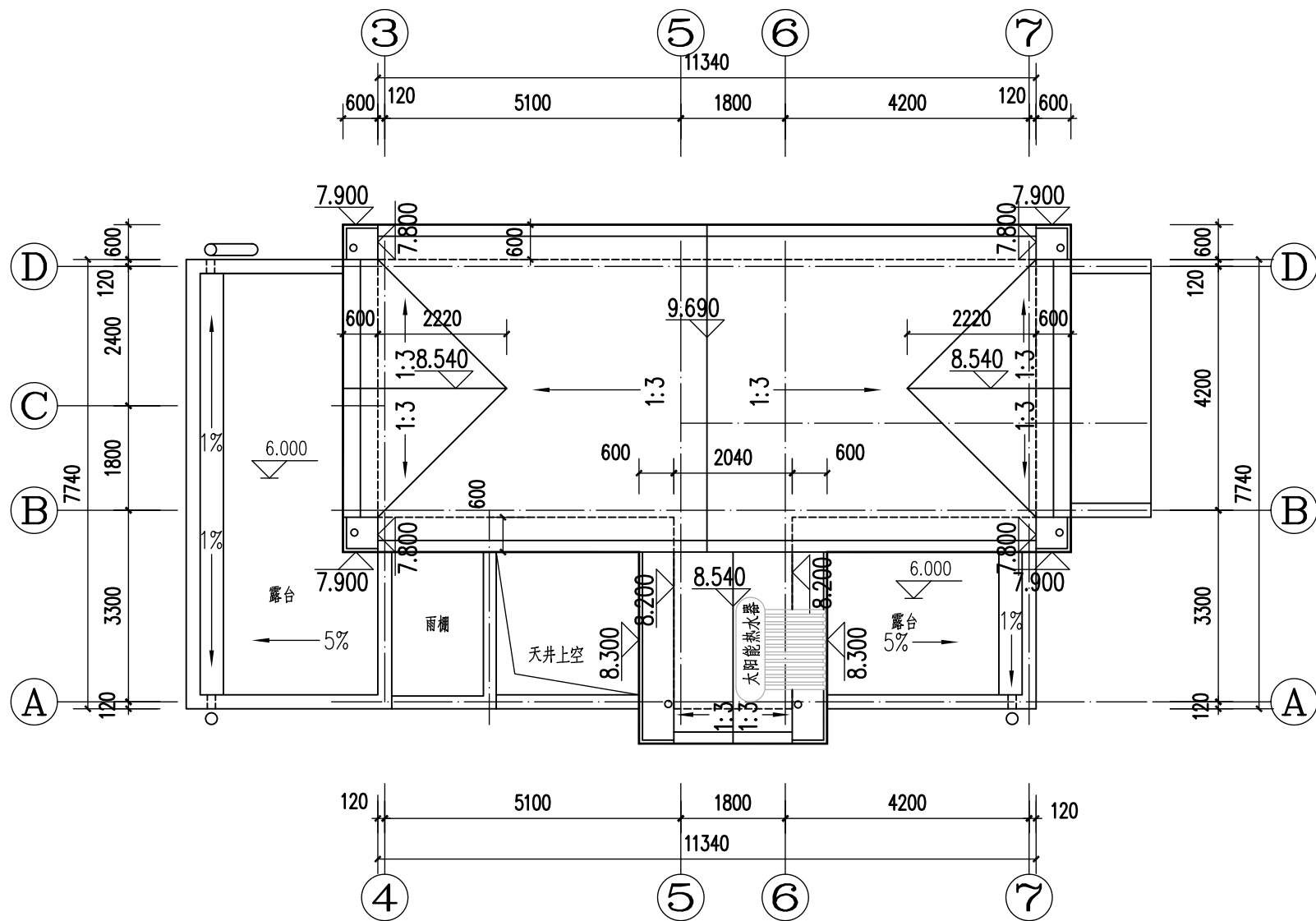
屋顶平面 1:100
