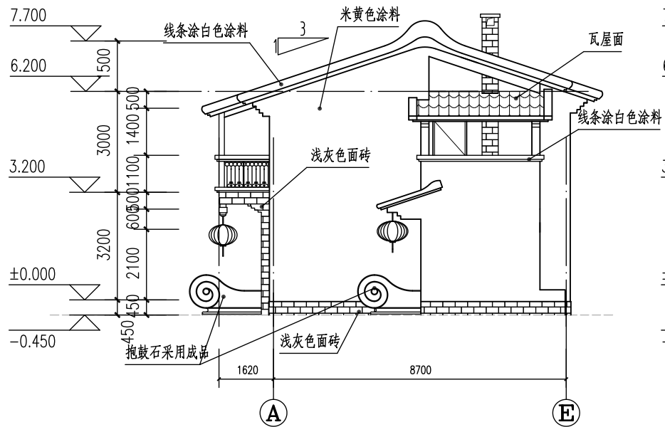
东立面 1:150
