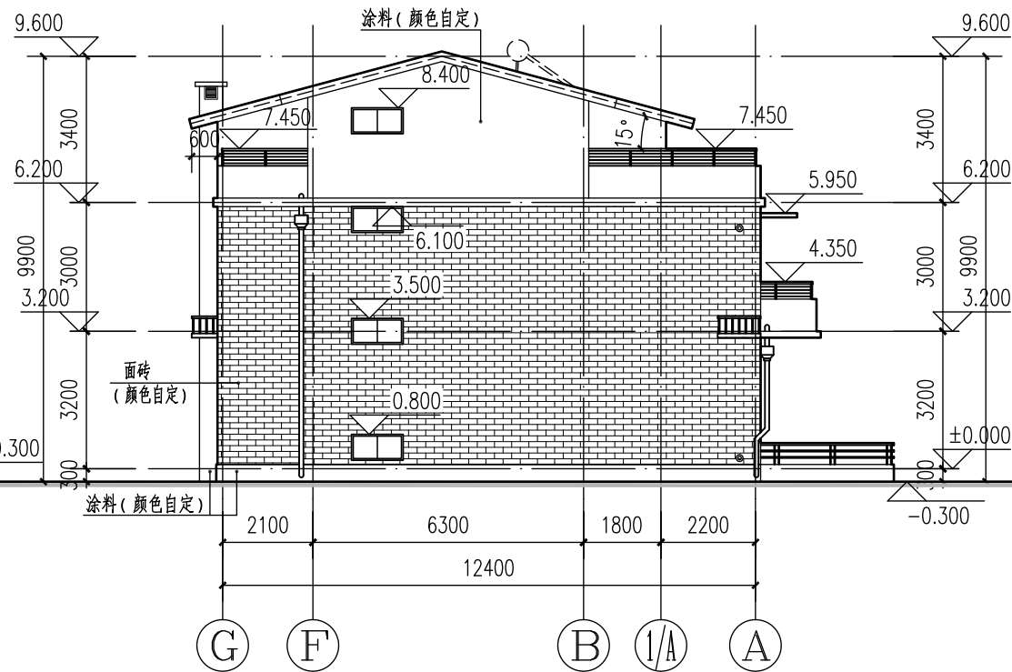
西立面图 1:150
