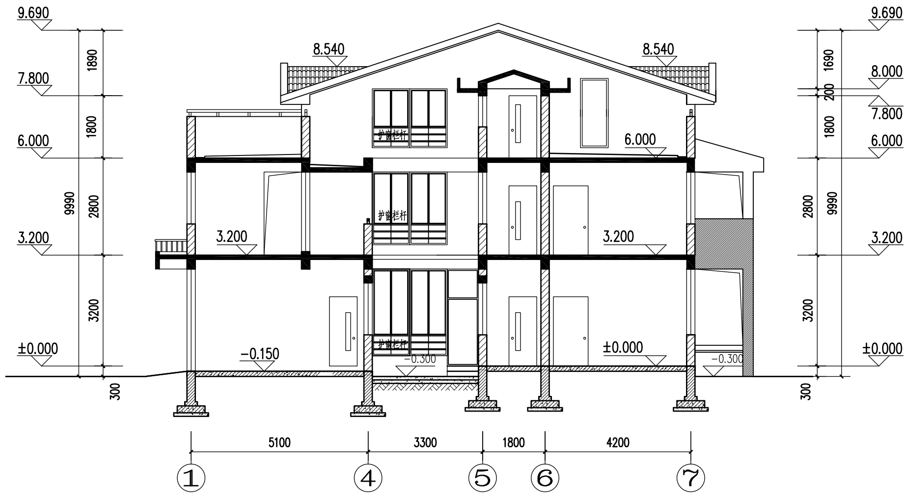
1-1剖面图 1:100
