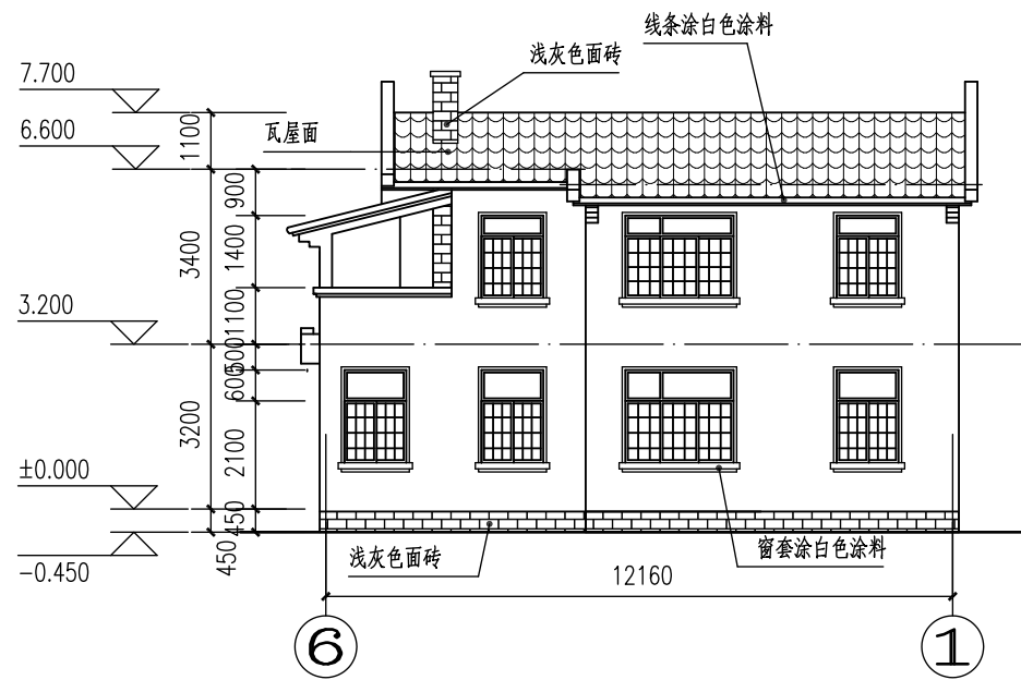
北立面 1:150
