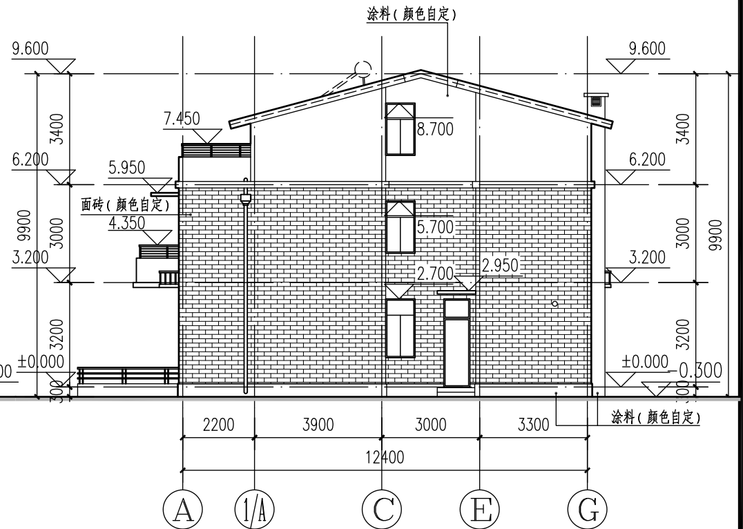
东立面图 1:150
