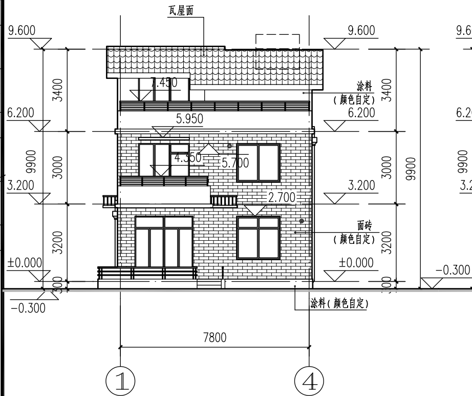
南立面图 1:150
