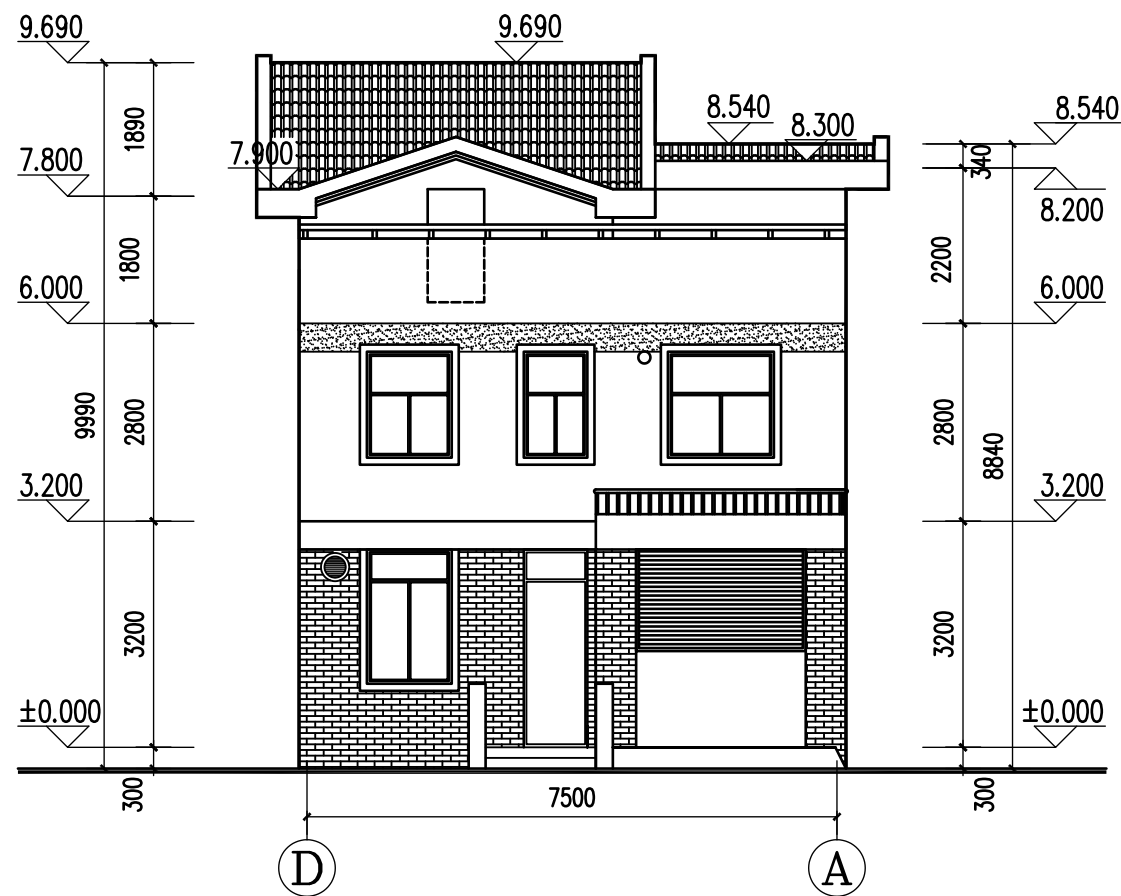
①② 北面图 1:100
