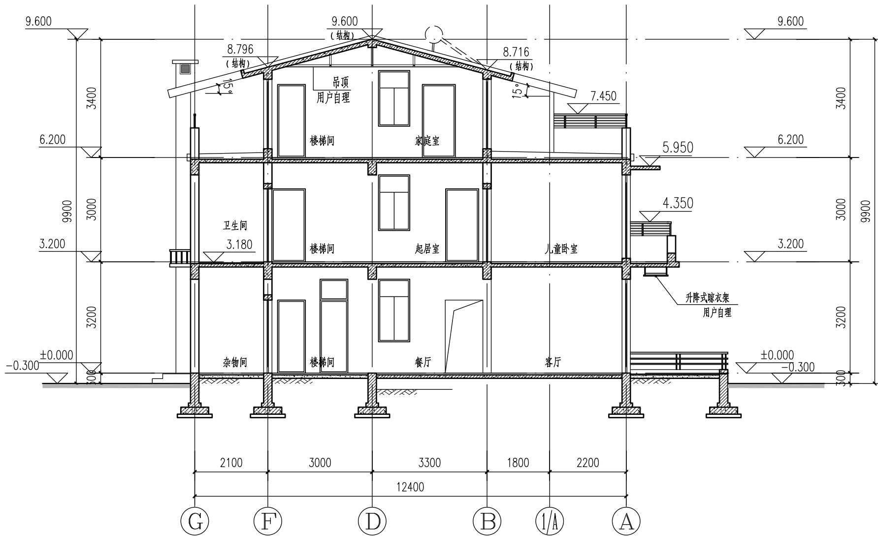
2-2剖面图 1:100
