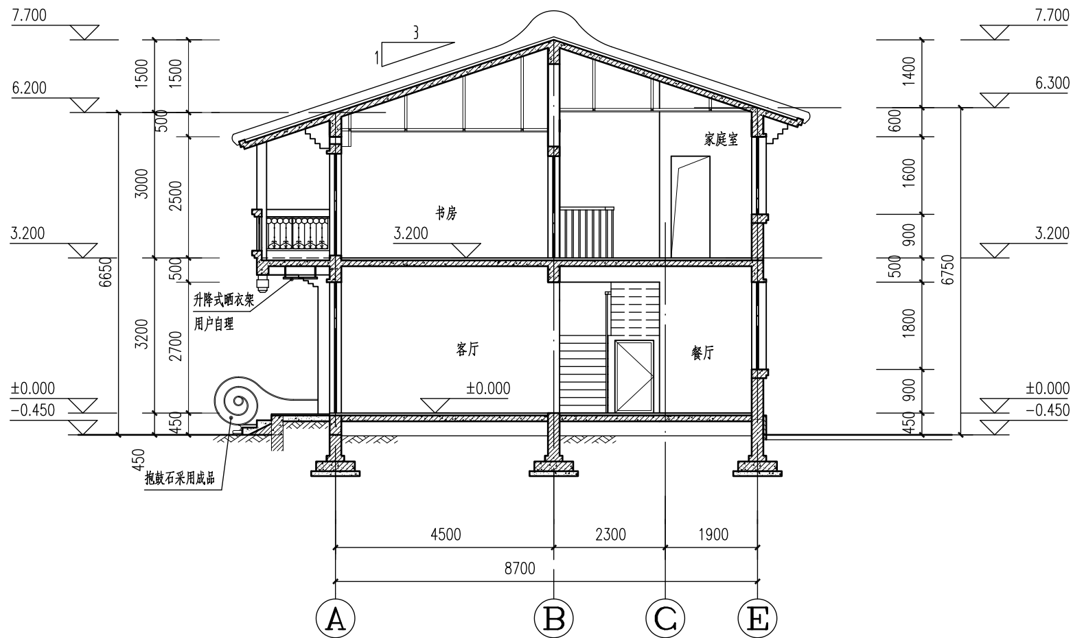
1-1剖面 1:100
