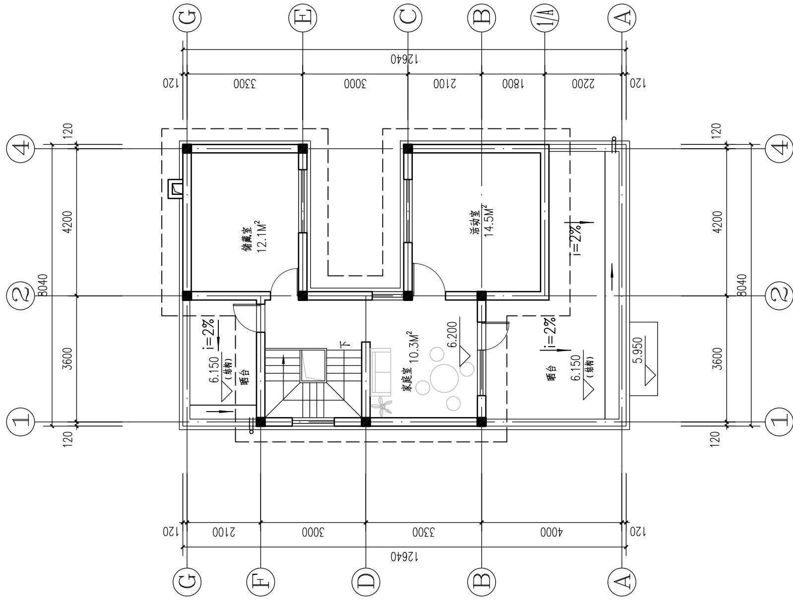
阁楼层平面
