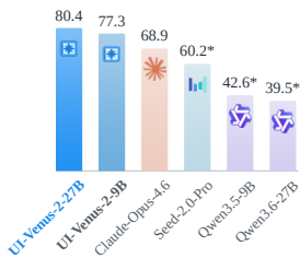
Odysseys
