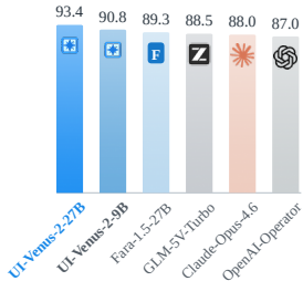
WebVoyager
