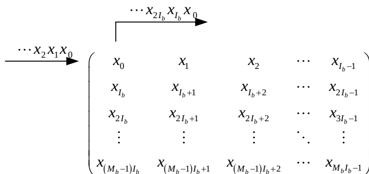
图10 比特交织
