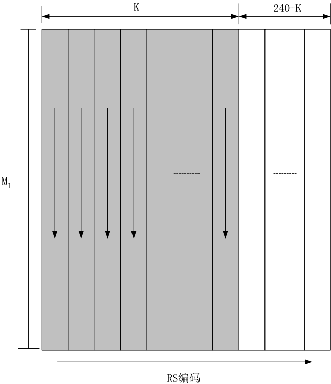
图9 字节交织器与 RS (240, K) 编码
