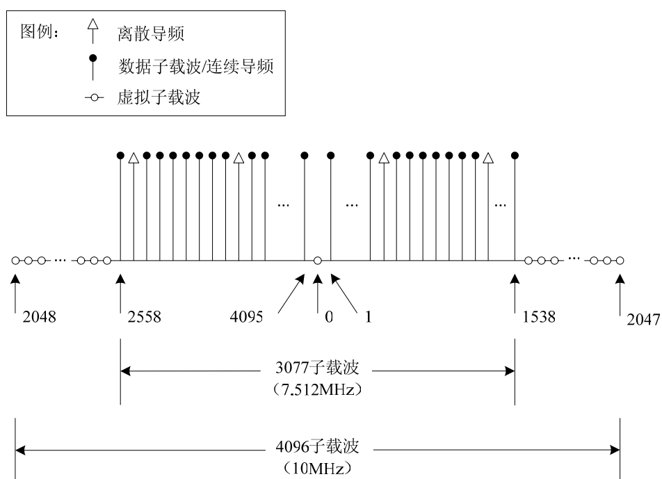
图16 OFDM 符号子载波结构示意图 ( B_f=8\text{MHz} )
