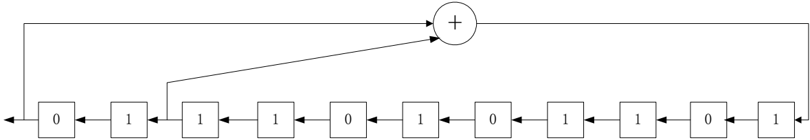
图5 同步信号伪随机序列生成器
