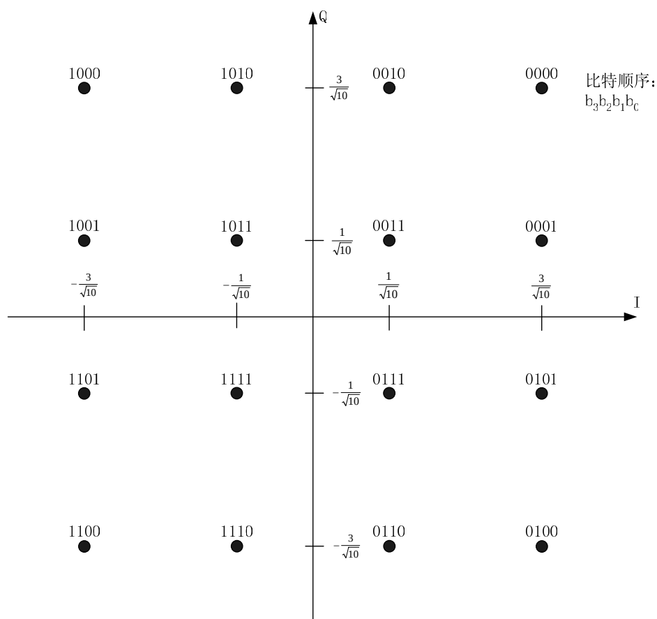
图13 16QAM 星座映射
