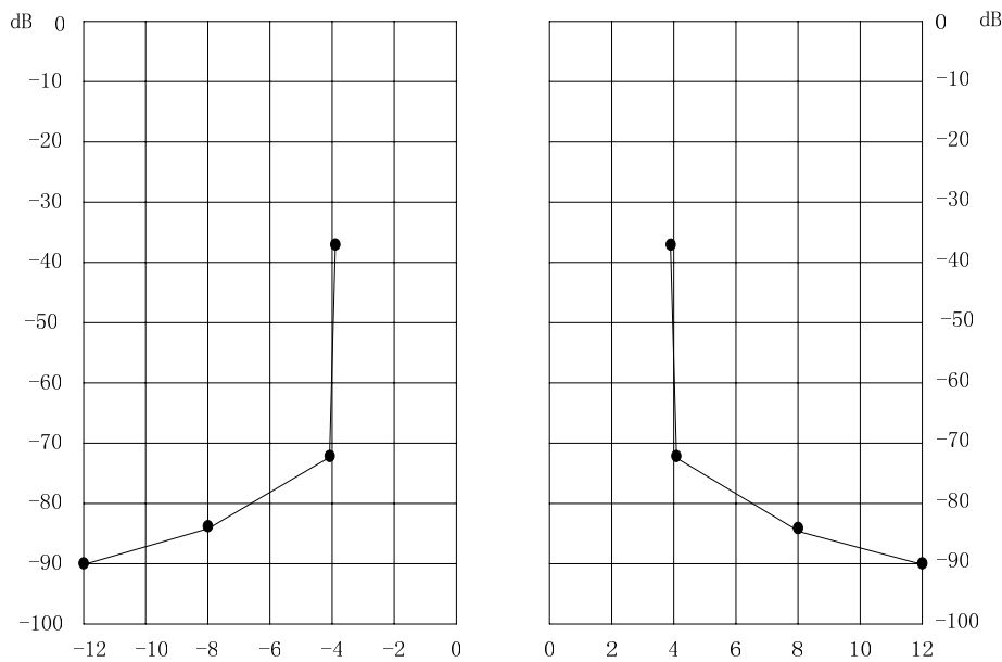
图20 调制信号频谱模板 ( B_f=8\text{MHz} )
