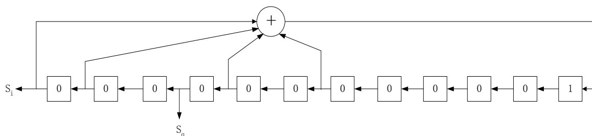
图15 产生扰码的线性反馈移位寄存器
