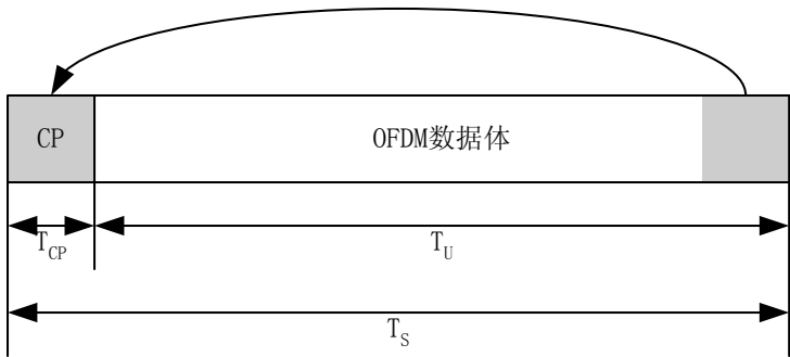
图6 OFDM 符号
