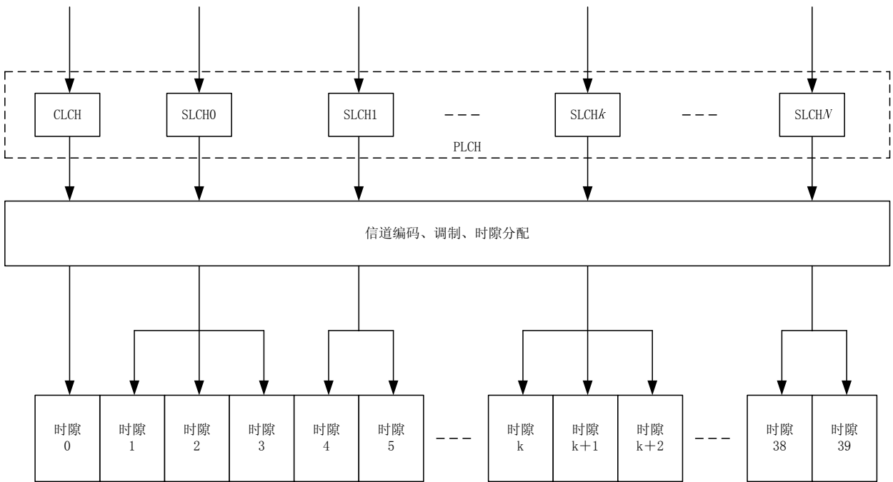
图1 移动多媒体广播系统广播信道物理层逻辑信道
