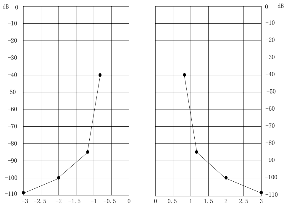
图21 调制信号频谱模板 (B f =2MHz)
