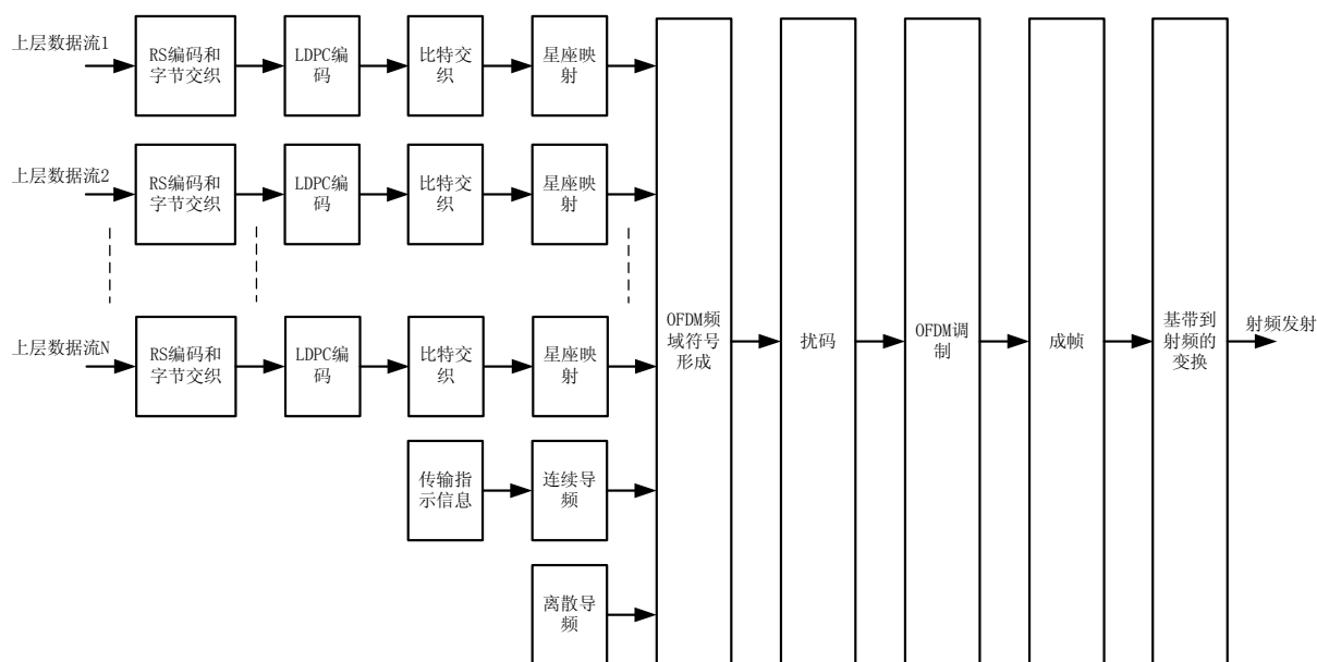
图2 物理层功能框图
