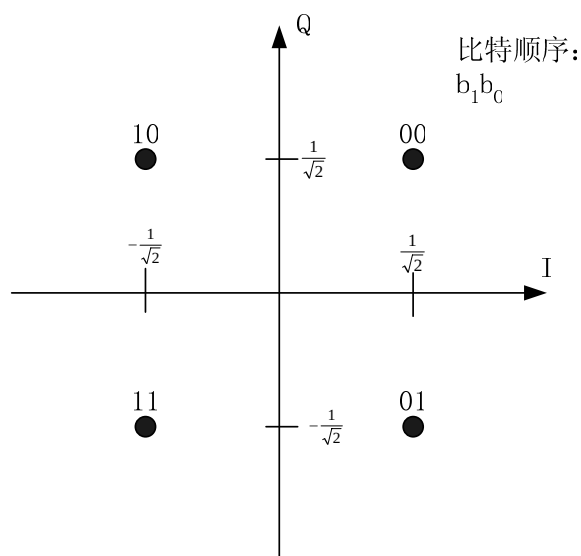
图12 QPSK 星座映射
