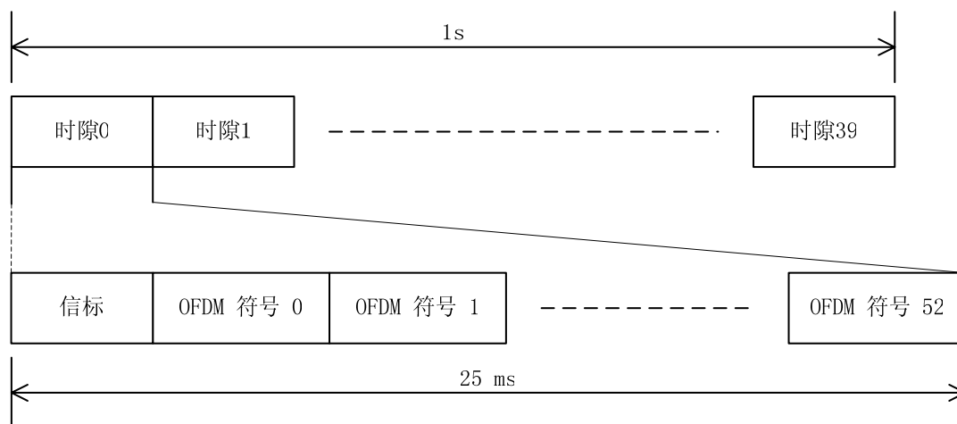
图3 基于时隙划分的帧结构
