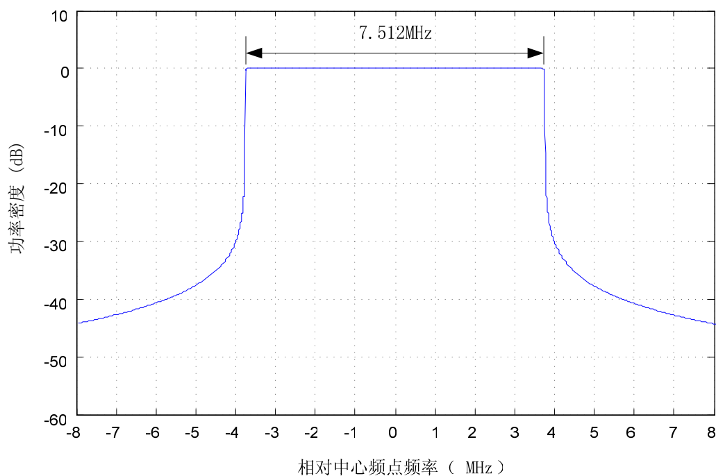
图18 广播信道调制信号理论功率谱 ( B_f=8\text{MHz} )
