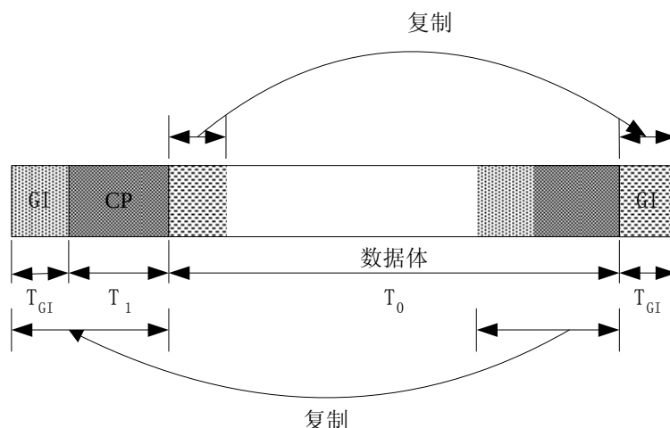
图8 保护间隔信号选取
