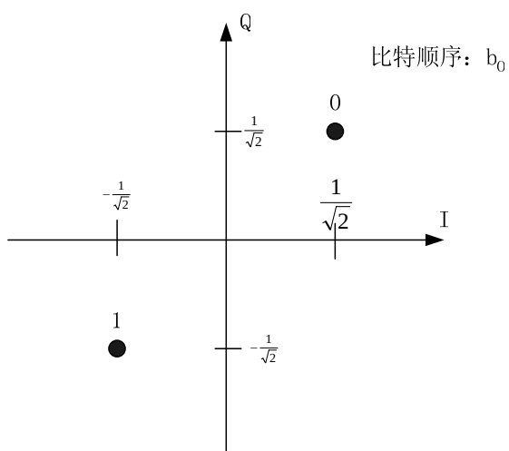
图11 BPSK 星座映射
