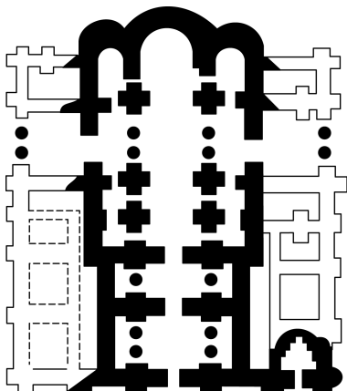
Десятинная церковь в Киеве (конец X в.) — образец крестовокупольного храма. План раскопанного фундамента
