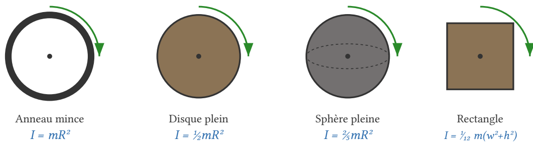
Figure 3: Moments d'inertie pour des formes courantes autour de leur centre. Notez comment la masse répartie loin de l'axe (anneau) donne un I plus grand que la masse concentrée au centre (disque).
