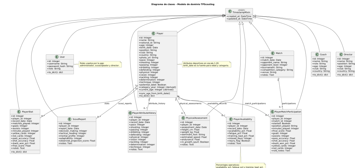
FIGURA 4-2. DIAGRAMA DE CLASES DEL MODELO DE DOMINIO.
