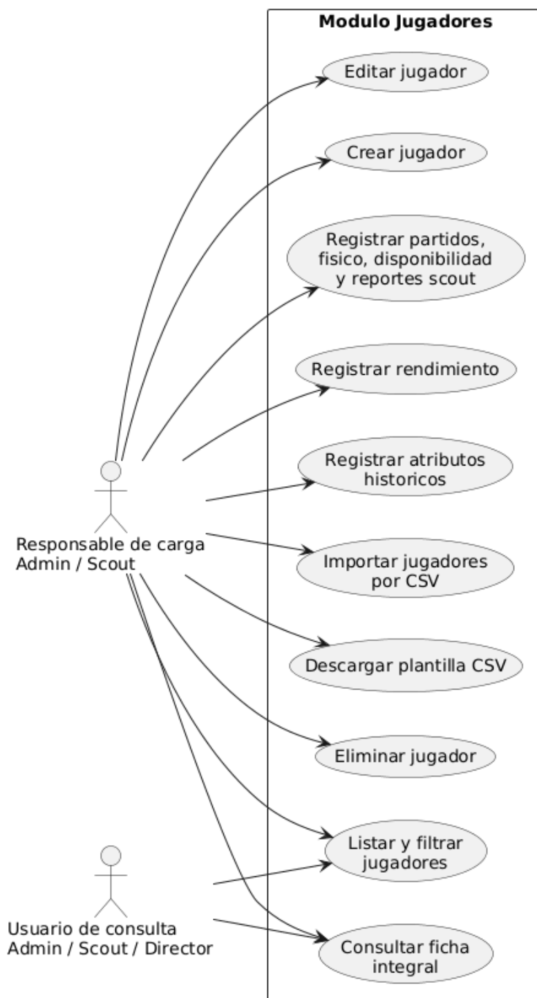
FIGURA 10-8. DIAGRAMA DE CASOS DE USO DE GESTIÓN DE JUGADORES AMPLIADO.
