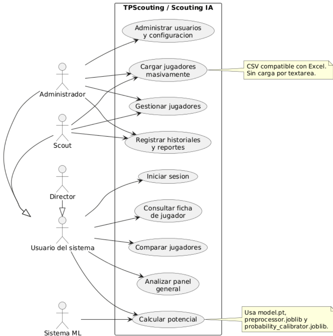
Diagrama de casos de uso - Vista general TPScouting
