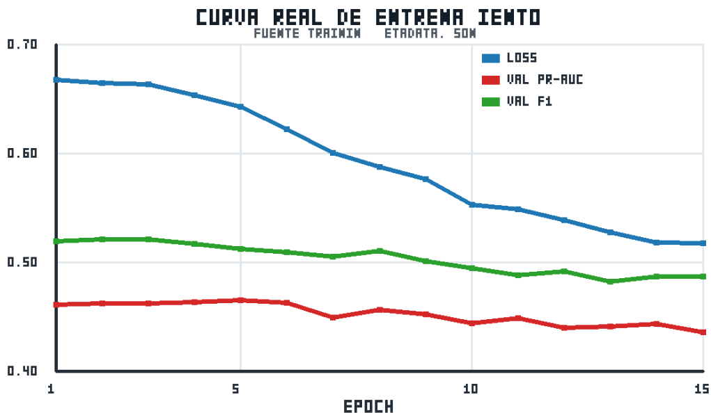
FIGURA 6-1. CURVA REAL DE ENTRENAMIENTO GENERADA DESDE TRAINING_METADATA.JSON.
