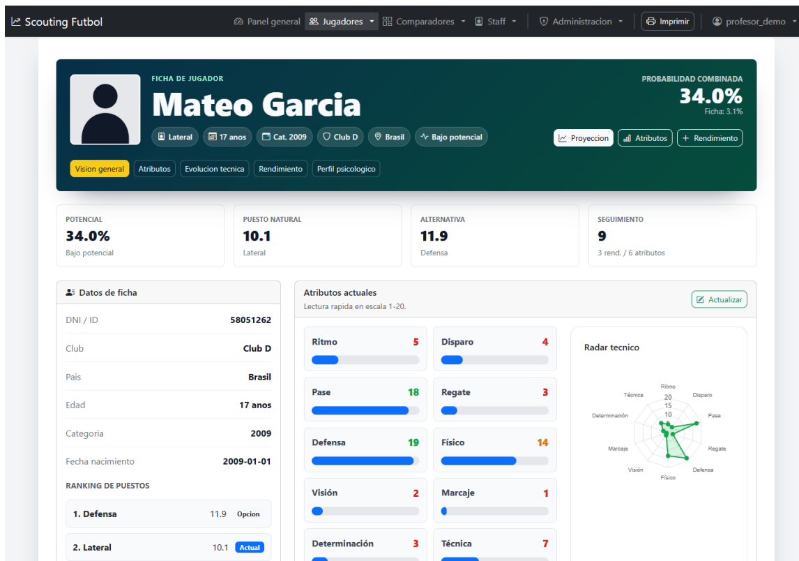
FIGURA 6-5. FICHA DE JUGADOR CON HISTORIAL, ATRIBUTOS Y ACCIONES CRUD EN MODALES.
