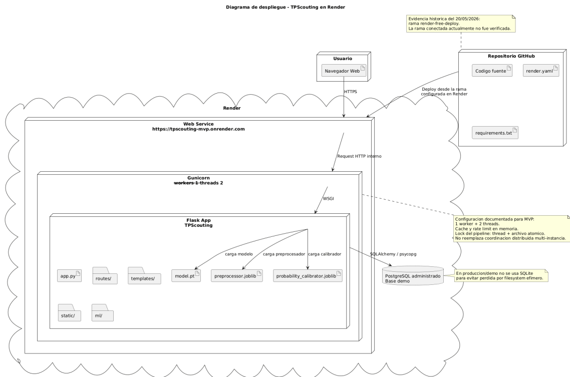
FIGURA 10-6. DIAGRAMA DE DESPLIEGUE EN RENDER AMPLIADO.
