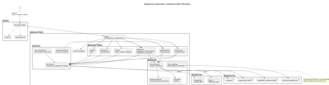
FIGURA 10-2. DIAGRAMA DE COMPONENTES DE TPSCOUTING AMPLIADO.
