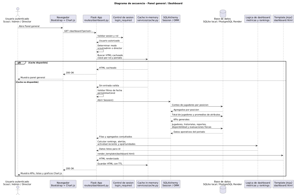
FIGURA 10-5. DIAGRAMA DE SECUENCIA DEL PANEL GENERAL AMPLIADO.
