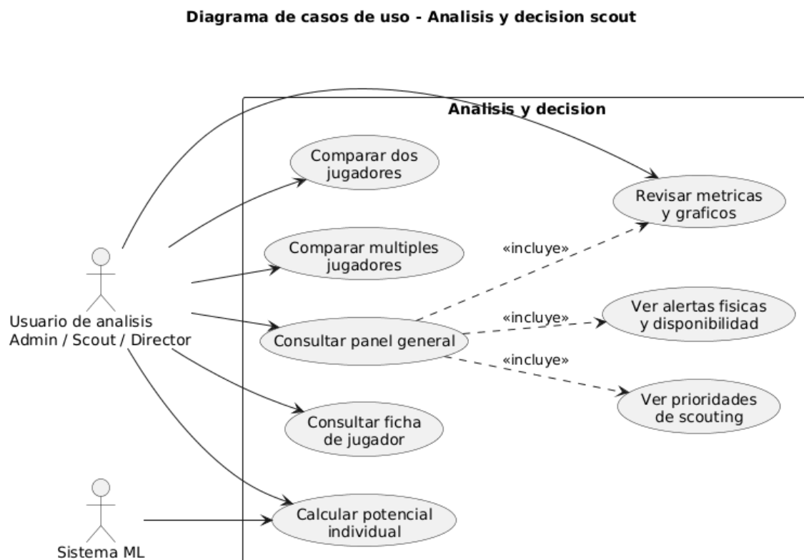
FIGURA 10-9. DIAGRAMA DE CASOS DE USO DE ANÁLISIS Y DECISIÓN SCOUT AMPLIADO.
