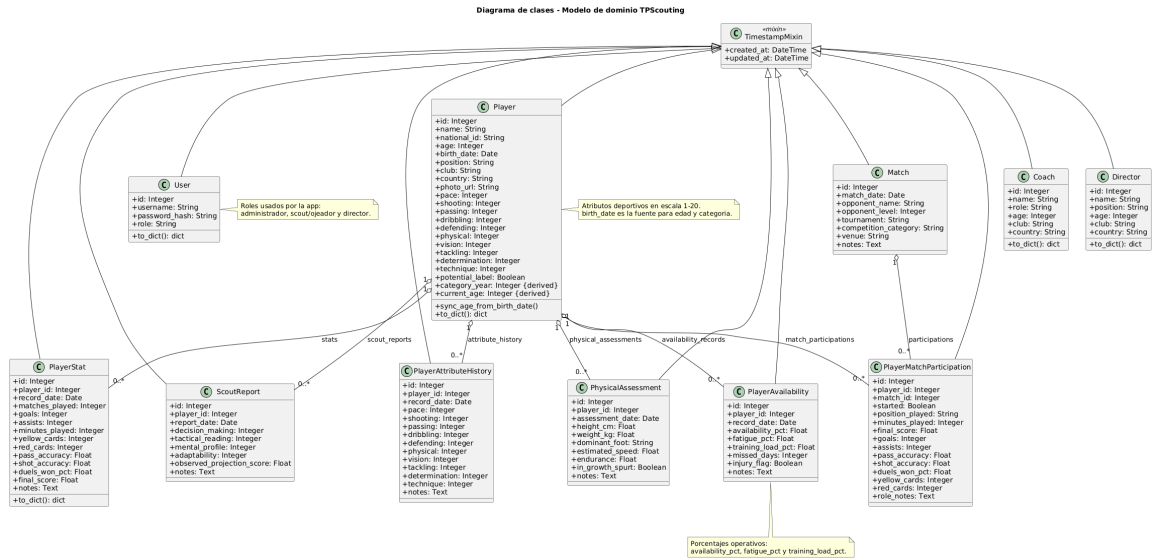
FIGURA 10-3. DIAGRAMA DE CLASES DEL MODELO DE DOMINIO AMPLIADO.
