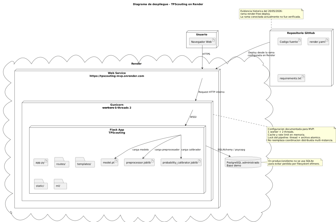
FIGURA 5-3. ARQUITECTURA DE DESPLIEGUE EN RENDER Y MECANISMOS OPERATIVOS DEL MVP.
