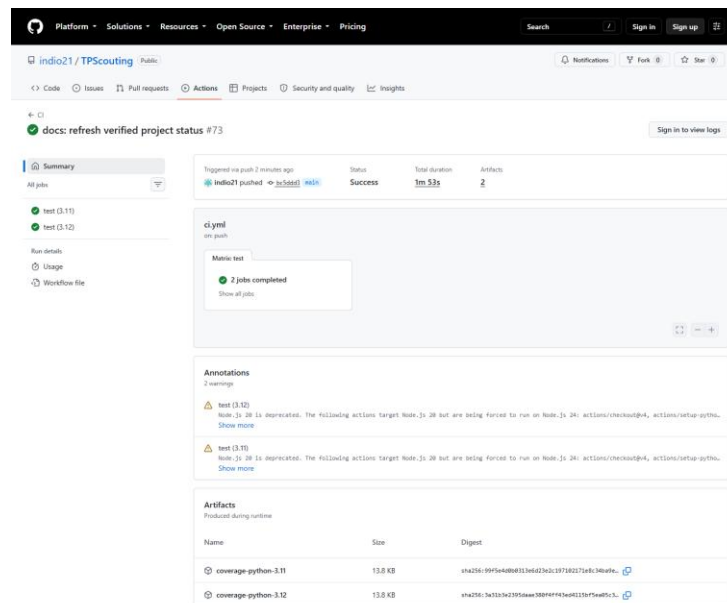
FIGURA 10-1. EVIDENCIA HISTÓRICA DE LA CI #73 DEL REPOSITORIO DE DESARROLLO.
