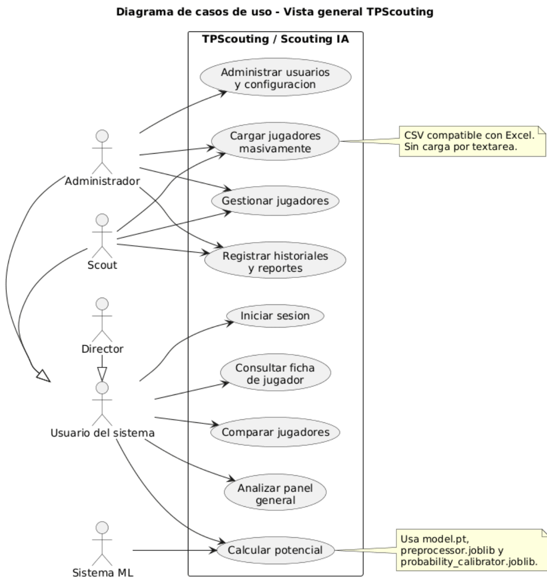
FIGURA 10-7. DIAGRAMA DE CASOS DE USO GENERAL AMPLIADO.
