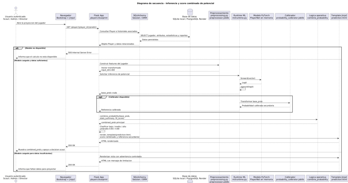
FIGURA 10-4. DIAGRAMA DE SECUENCIA DE INFERENCIA AMPLIADO.
