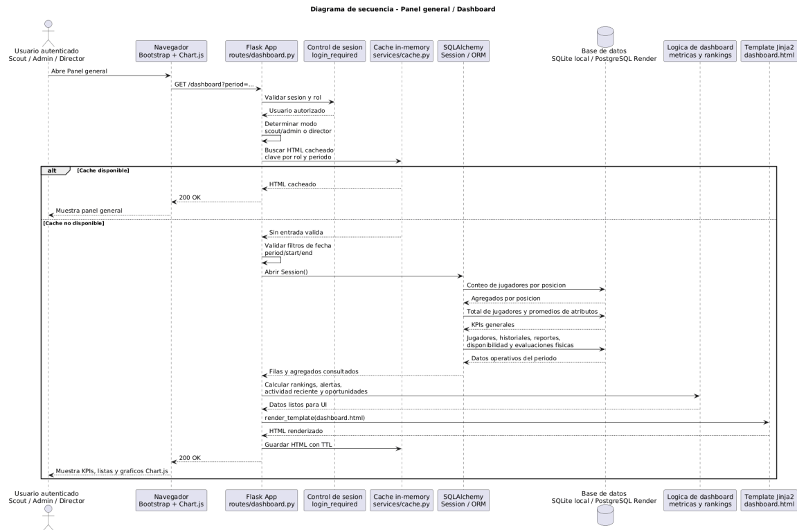
FIGURA 5-2. SECUENCIA DE CARGA DEL PANEL GENERAL.
