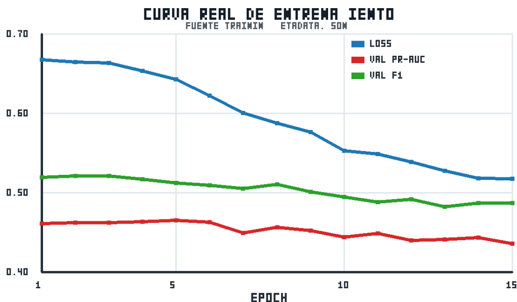
FIGURA 6-1. CURVA REAL DE ENTRENAMIENTO GENERADA DESDE TRAINING_METADATA.JSON.
