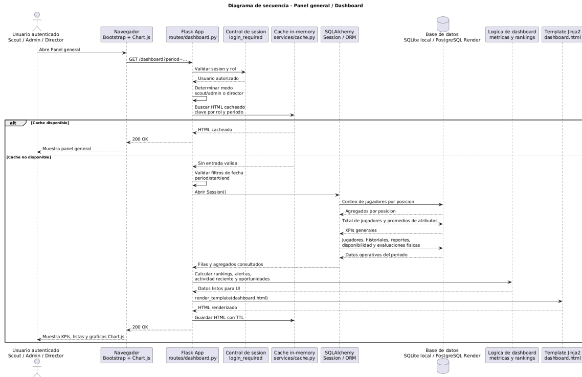
FIGURA 10-5. DIAGRAMA DE SECUENCIA DEL PANEL GENERAL AMPLIADO.
