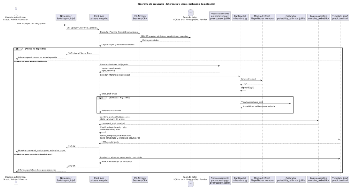
FIGURA 10-4. DIAGRAMA DE SECUENCIA DE INFERENCIA AMPLIADO.
