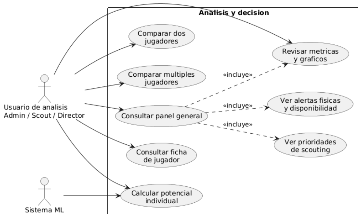
FIGURA 10-9. DIAGRAMA DE CASOS DE USO DE ANÁLISIS Y DECISIÓN SCOUT AMPLIADO.
