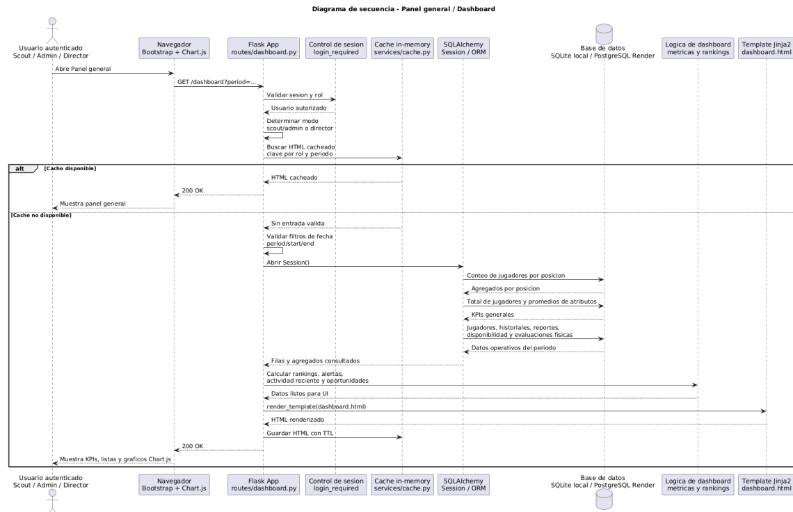
FIGURA 5-2. SECUENCIA DE CARGA DEL PANEL GENERAL.
