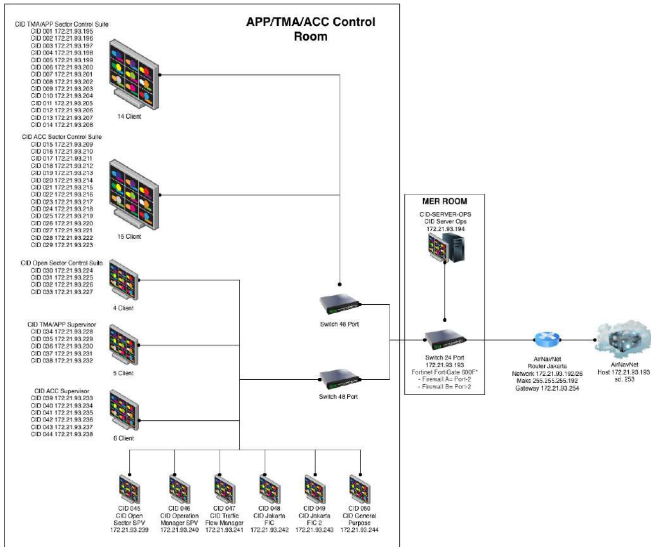
Gambar 3. Topologi Jaringan CID AirNav Cabang JATSC
