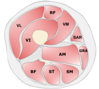
schéma d'une coupe de cuisses
