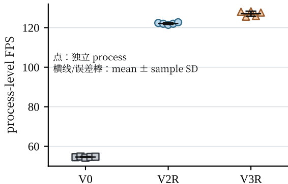
(a) 5 次独立进程 FPS
