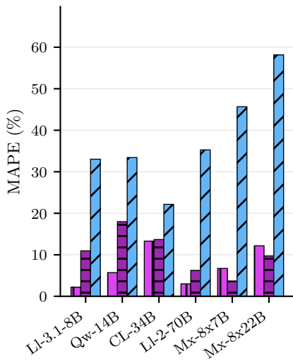
E2E Mean
