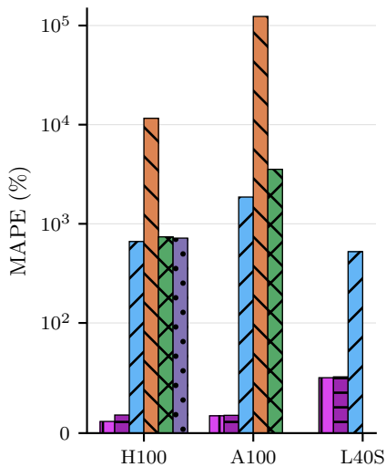
TTFT Mean
