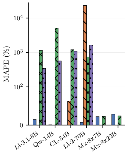
TTFT Mean
