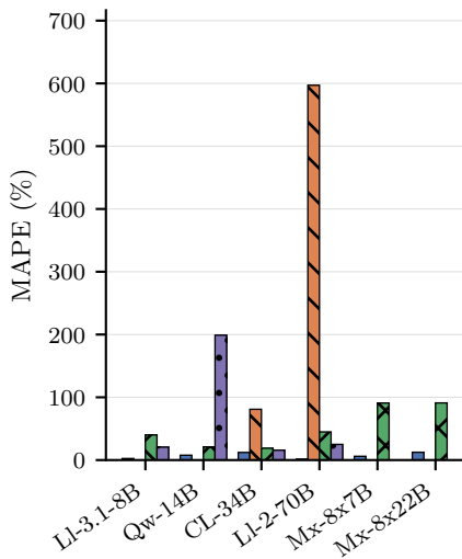
E2E Mean
