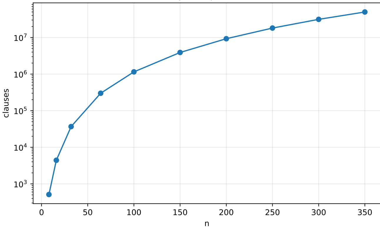
Encoding size, pairwise AMO
