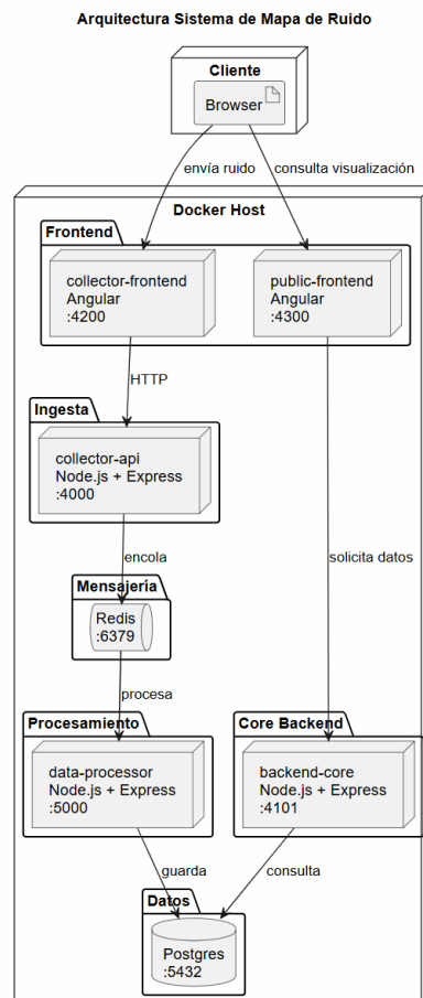
Figura 3. Diagrama de despliegue
