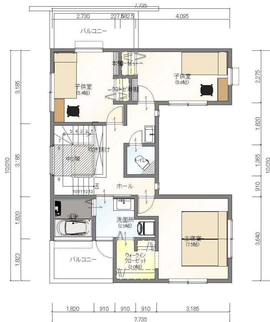
2階平面図
