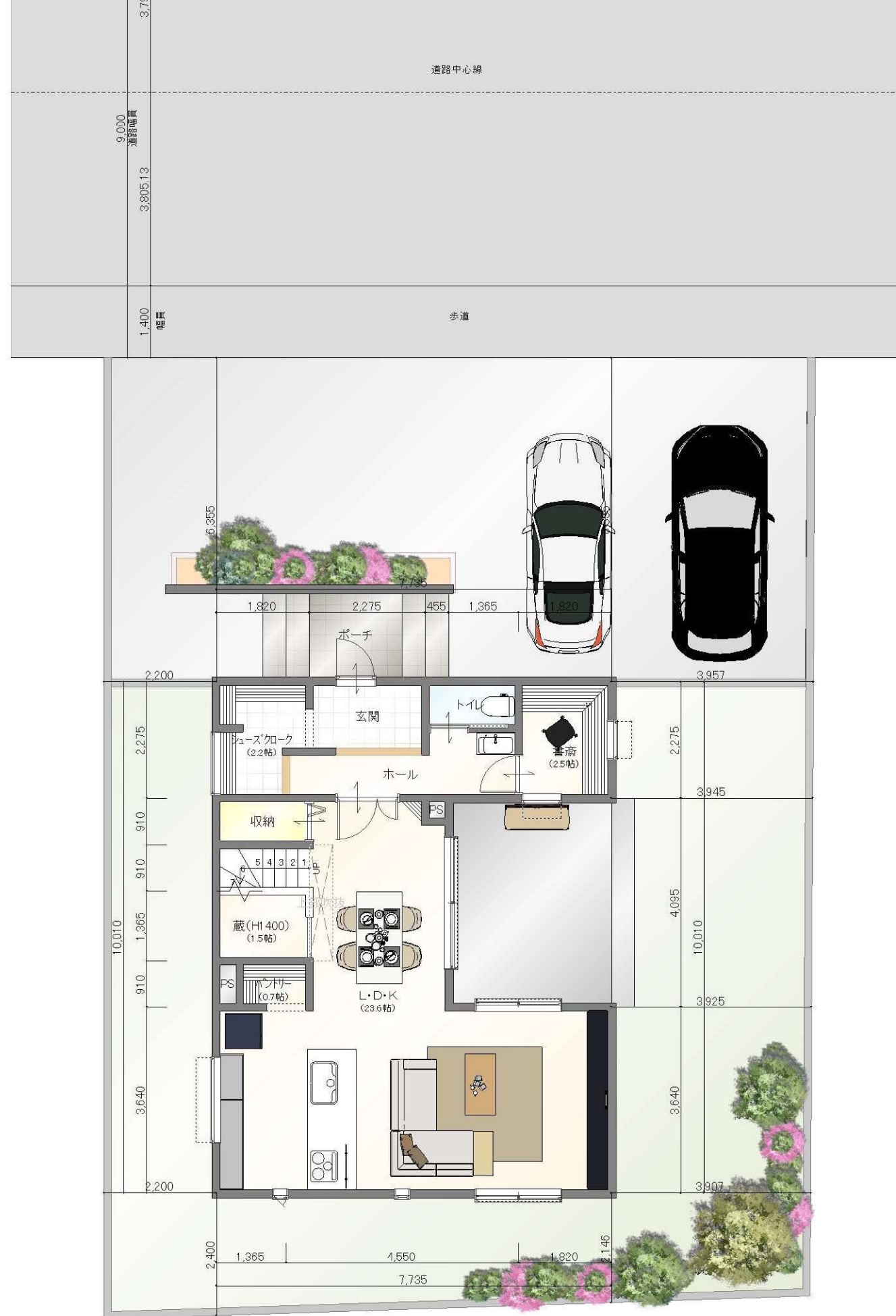
配置図
