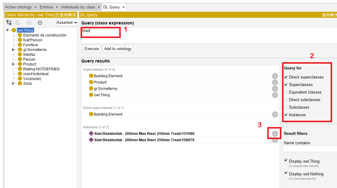
Figura 8: Ejemplo de consulta DL en Protégé.
