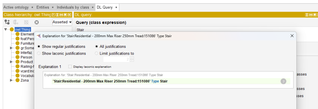
Figura 9: Ejemplo de explicación ofrecida por el razonador.
