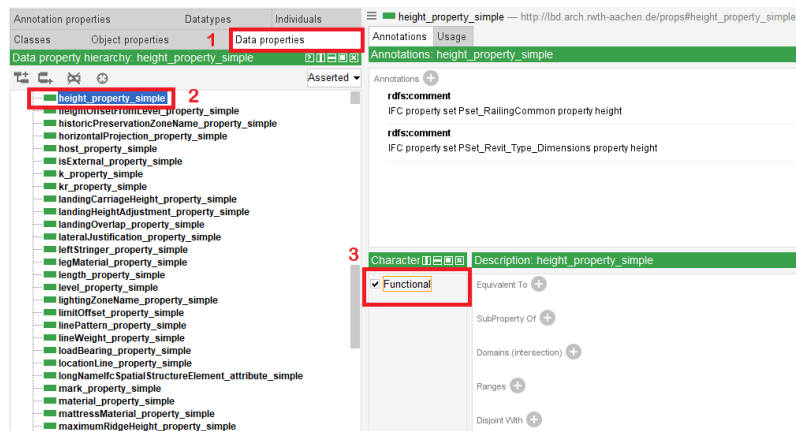
Figura 11: Marcar la propiedad como funcional.
