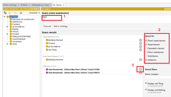
Figura 9: Ejemplo de consulta DL en Protégé.
