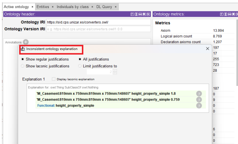
Figura 14: Explicación de la inconsistencia generada.
