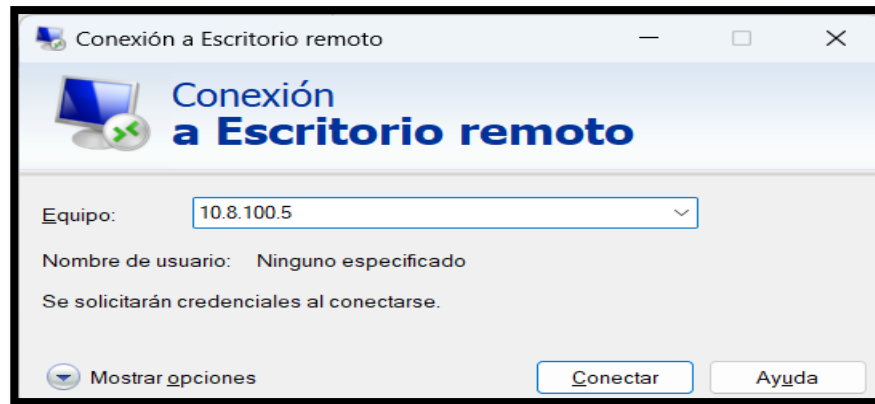
Imagen 11. Escritorio remoto
