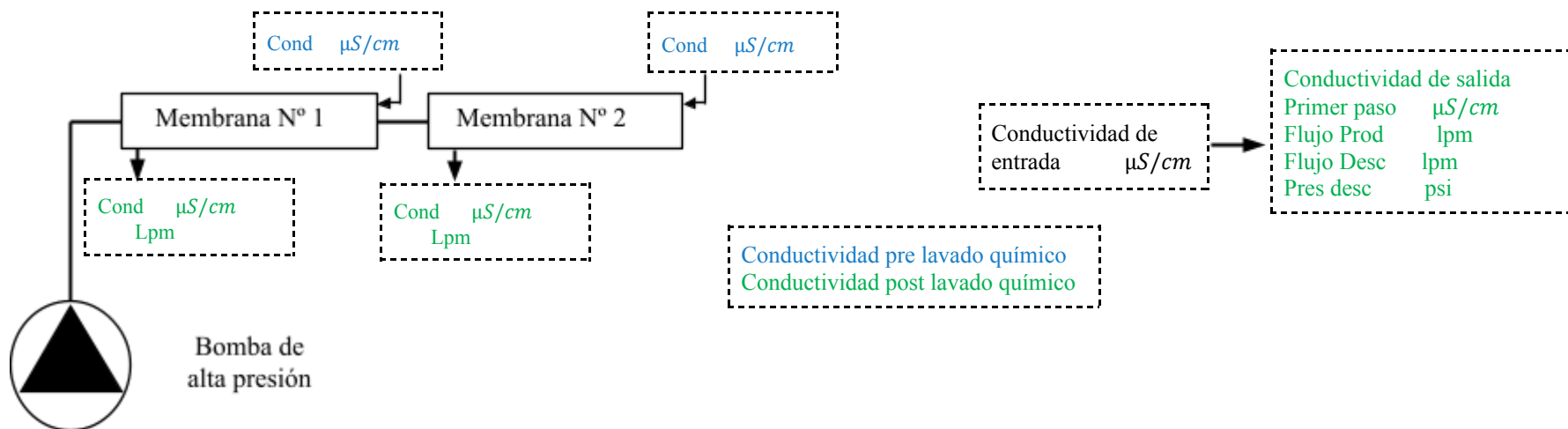
Configuración de las membranas de la Osmosis Reversa 1
