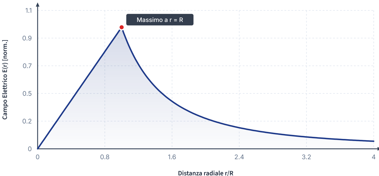
Andamento del Campo Elettrico E(r) per Sfera Uniformemente Carica
