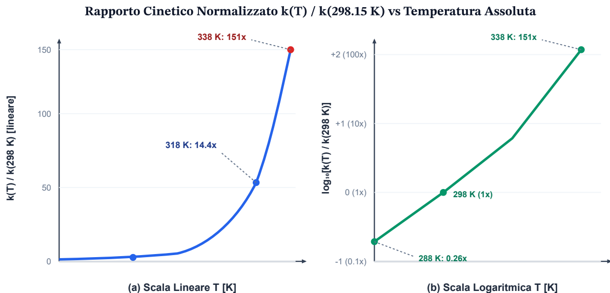
Grafico 2 — Risposta Dinamica di k(T) / k(298.15 \text{ K}) in funzione di T : (a) Scala Lineare per l'Esplosione Termica; (b) Scala Semilogaritmica per le Basse Temperature
