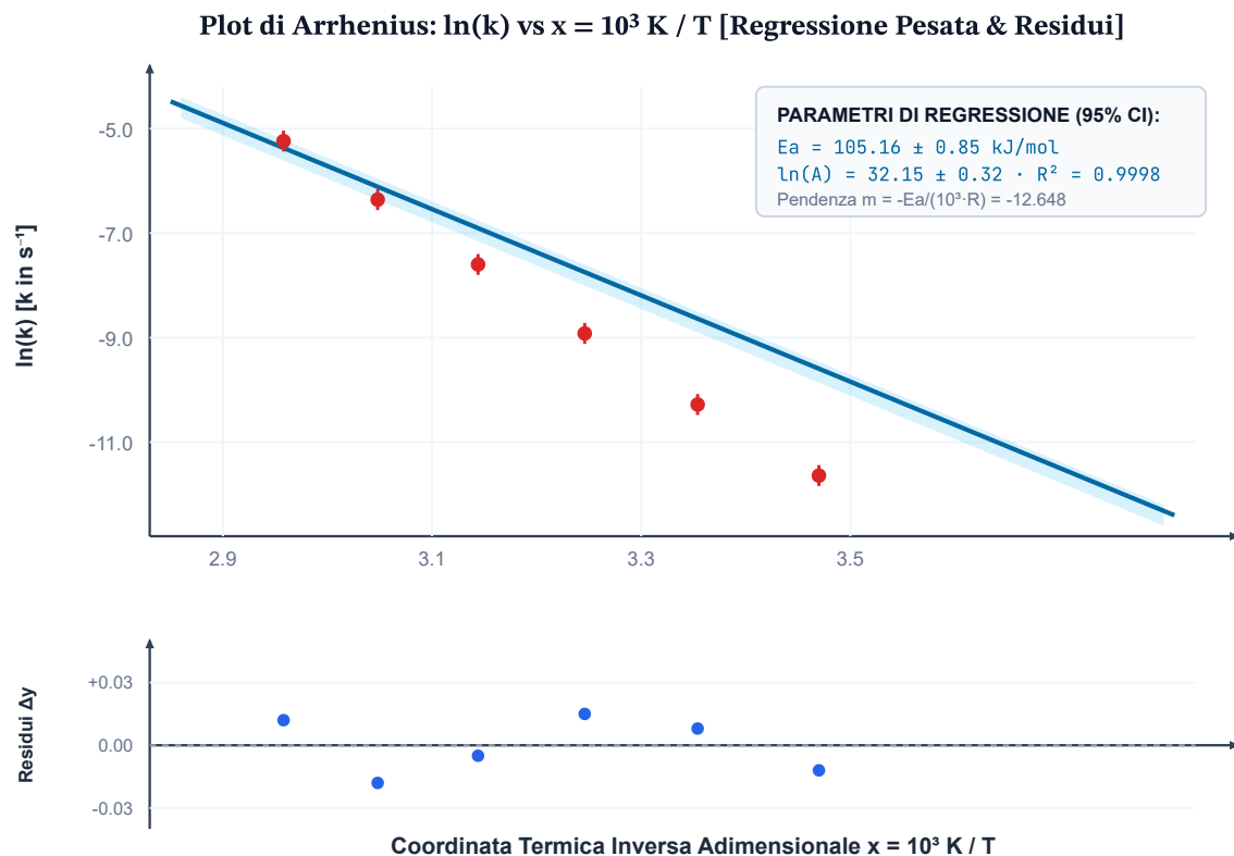
Grafico 1 — Trasformazione di Arrhenius a Due Pannelli: (a) Fit di Regressione con Banda di Confidenza 95%; (b) Grafico dei Residui
