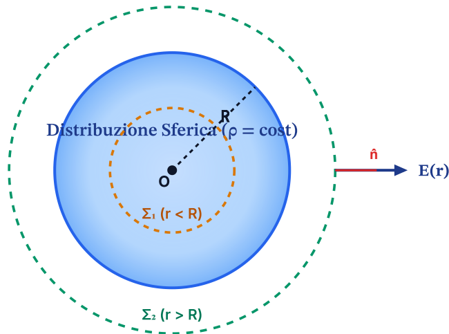
Figura 1: Schema Geometrico Quotato della Sfera Carica e Superfici Gaussiane Concentriche
