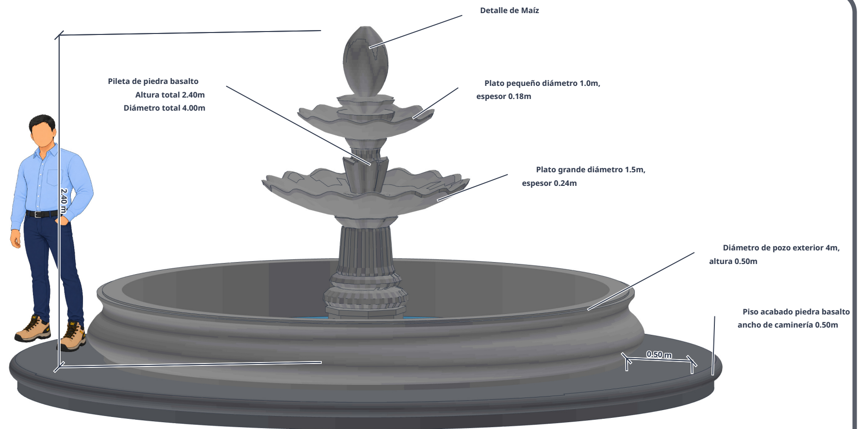
Vista 3D Pileta Ornamental
