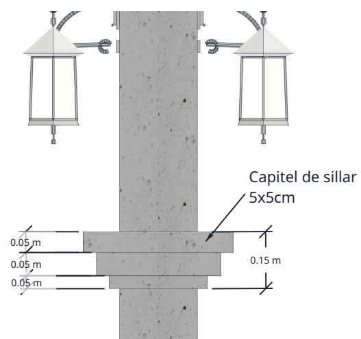
DETALLE DE CAPITEL DE SILLAR ESC. 1:20
