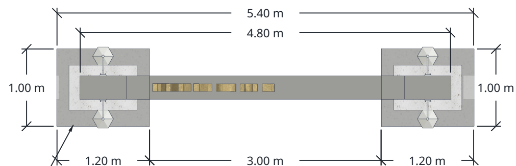
VISTA DE PLANTA ESC. 1:50
