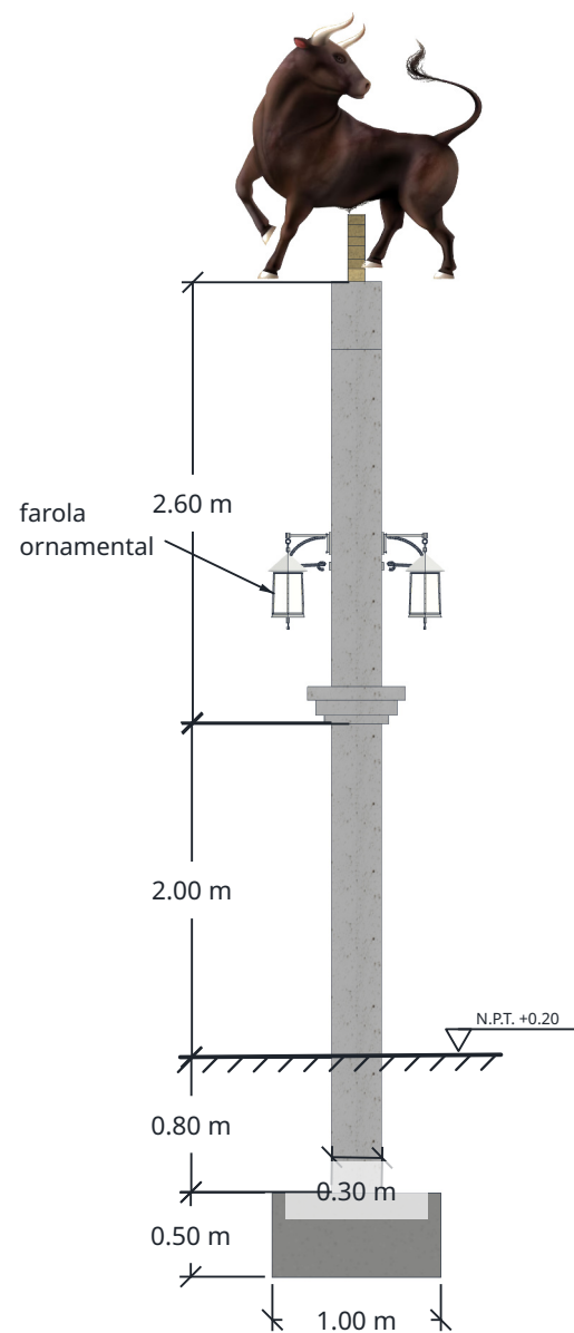
VISTA LADO DERECHO ESC. 1:50
