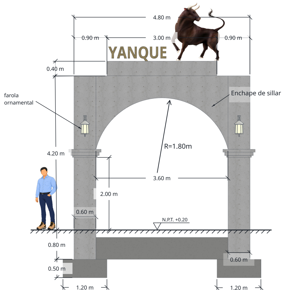
VISTA DE FRENTE ESC. 1:50
