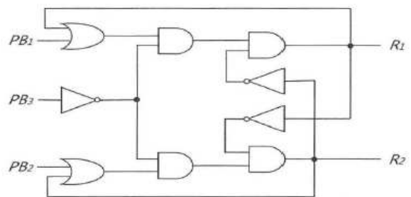
<가> 무접점 회로
