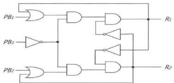
<가> 무접점 회로
