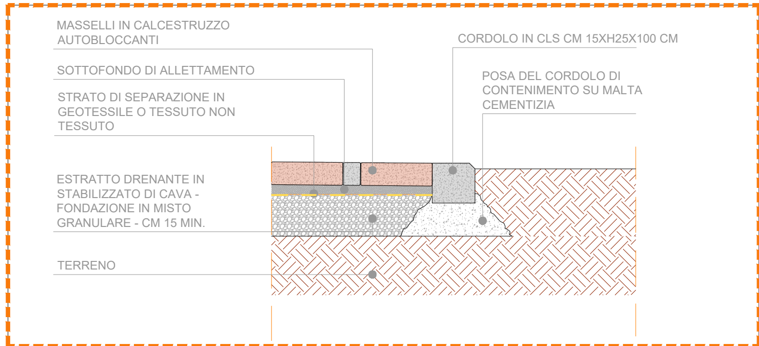
DETTAGLIO 1 - STRATIGRAFIA NUOVA PAVIMENTAZIONE IN AUTOBLOCCANTI
