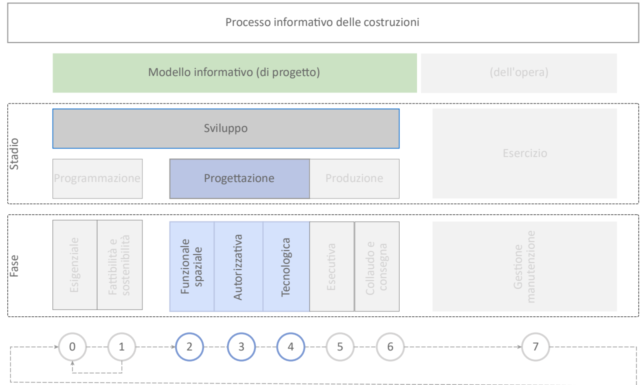
Figura 2 Processo informativo delle costruzioni (rielaborazione UNI 11337-1:2017) con evidenziati stadio e fasi oggetto del presente incarico.
