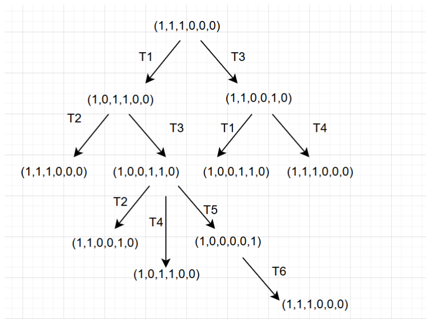
Рис. 2.2: Дерево достижимости
