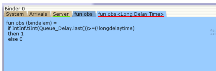
Рис. 2.14: Функция Observer монитора Long Delay Time
