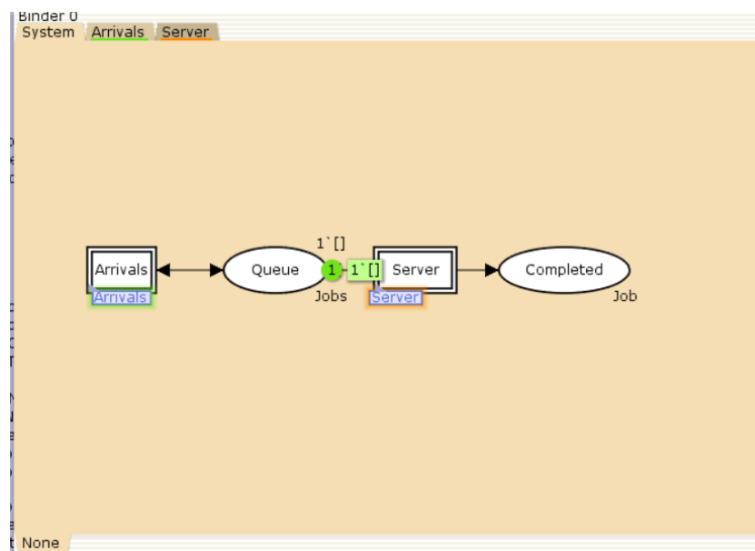
Рис. 2.5: Параметры элементов основного графа системы обработки заявок в очереди
