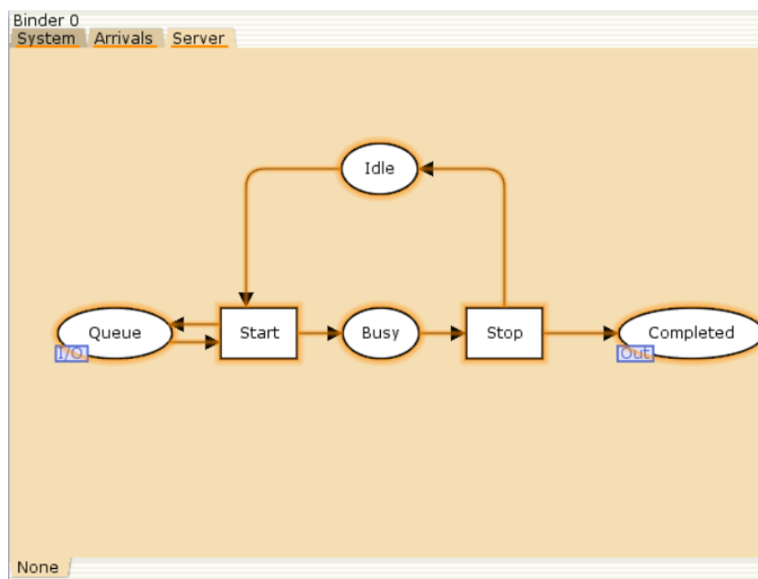
Рис. 2.3: Граф процесса обработки заявок на сервере системы
