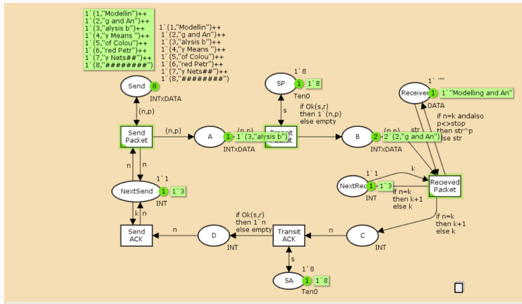
Рис. 6: Запуск модели простого протокола передачи данных
