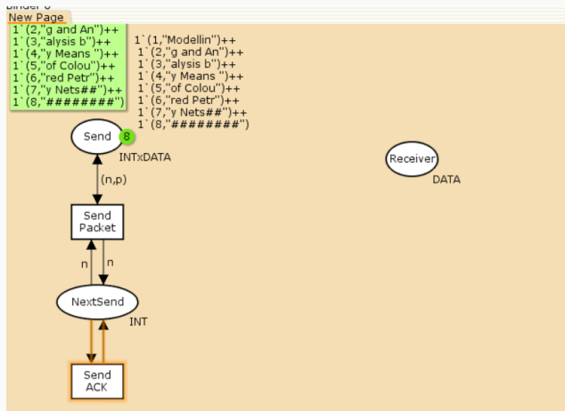
Рис. 2: Начальный граф
