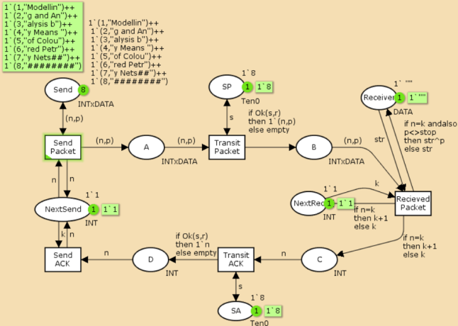
Рис. 5: Модель простого протокола передачи данных
