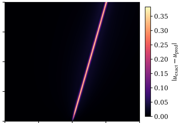
(b) |u_{\text{exact}} - u_{\text{TRG-PINN}}|
