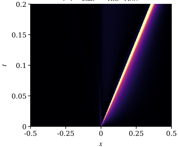
(d) |u_{\text{exact}} - u_{\text{TRG-PINN}}|
