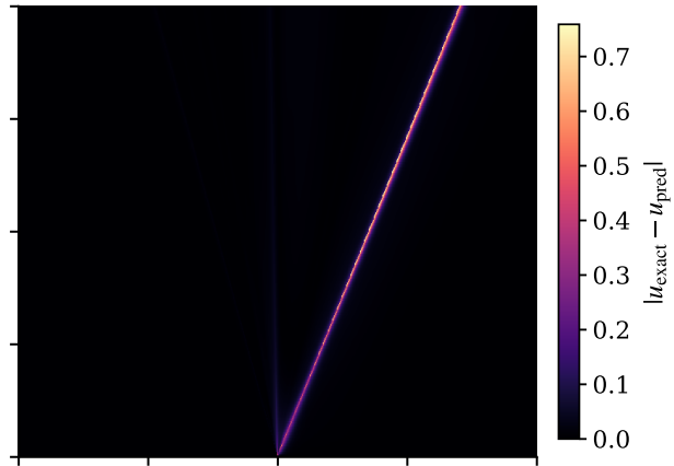
(e) |u_{\text{exact}} - u_{\text{TRG-PINN}}|
