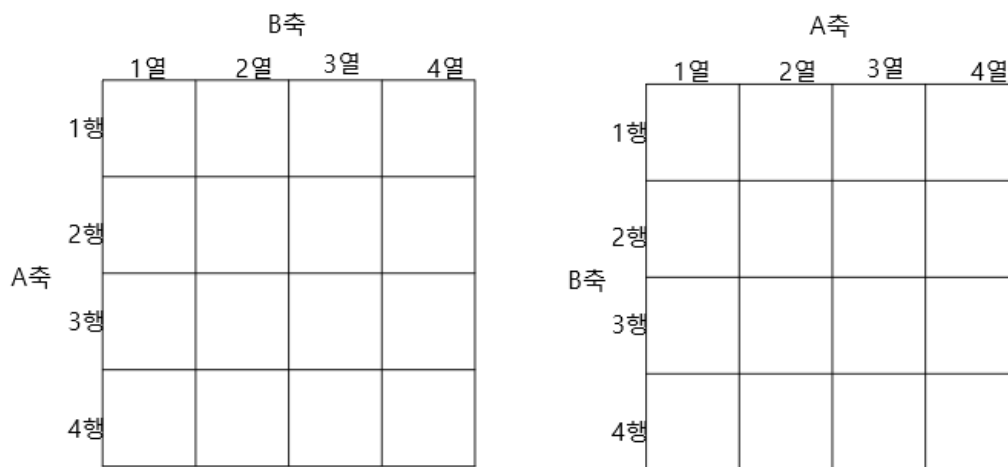
그림 5.5.1: 4×4 카르노맵 좌표계 — 행 번호는 위에서 아래로 1에서 4, 열 번호는 왼쪽에서 오른쪽으로 1에서 4
