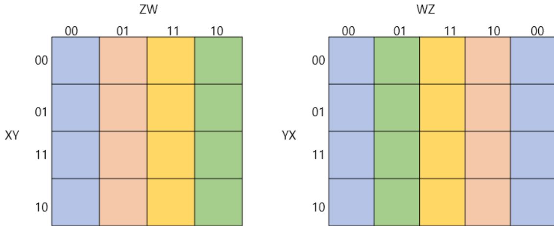
Figure 4: 표 5.5.3: 가로축의 변수 앞뒤 교환에 따른 상하역전관계를 색깔로 표현
