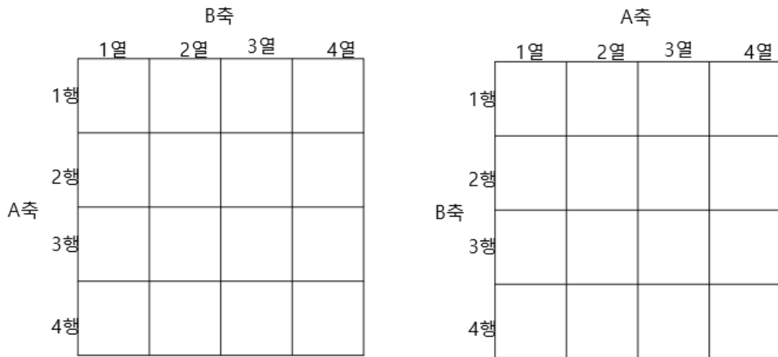
그림 5.5.1: 4×4 카르노맵 좌표계 – 행 번호는 위에서 아래로 1에서 4, 열 번호는 왼쪽에서 오른쪽으로 1에서 4 한편 카르노맵의 변수 배열은 일반적인 이진수 순서가 아닌 그레이코드 (Gray Code) 순서를 사용한다. 2변수 그레이코드의 배열 순서는 다음과 같다.
