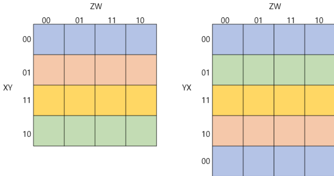
Figure 6: 그림 5.5.2: 세로축의 변수 앞뒤 교환에 따른 상하역전관계를 색깔로 표현
