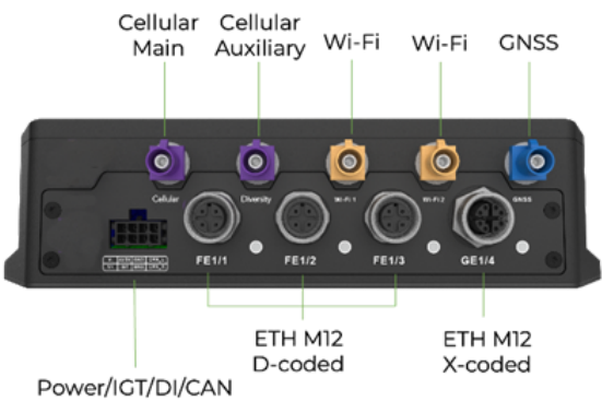
引脚接口图4G版本
