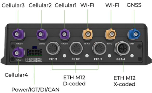
引脚接口图5G版本
