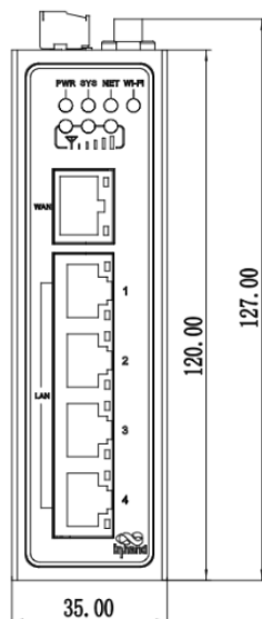
接口图
