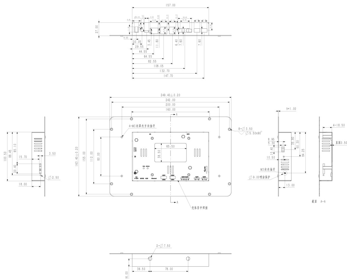
产品尺寸图
