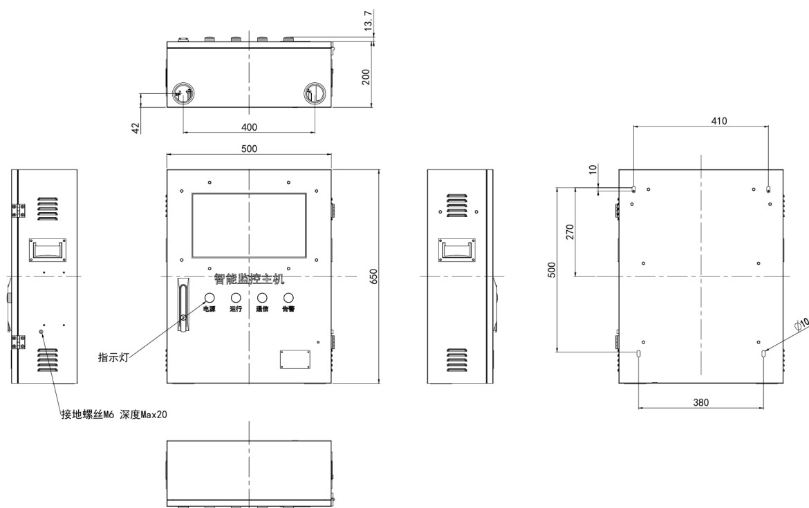
尺寸图
