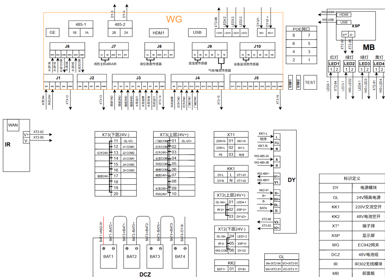
接线图
