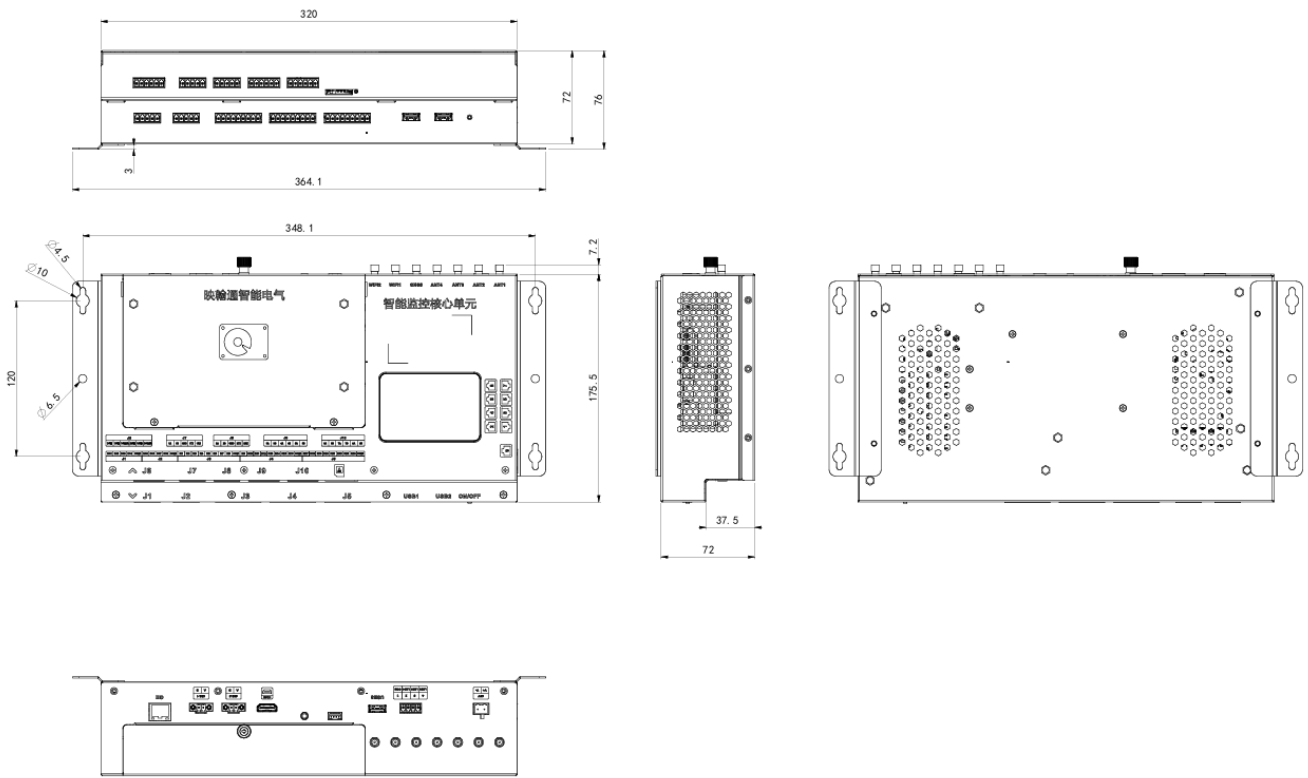
尺寸图
