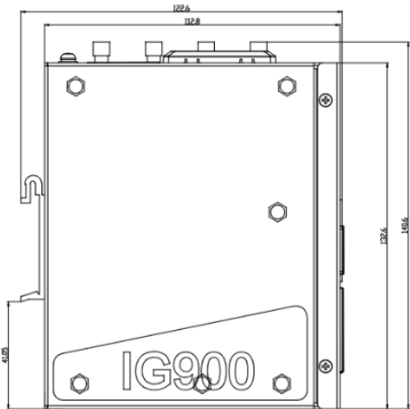
正视图
