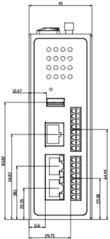
接口图
