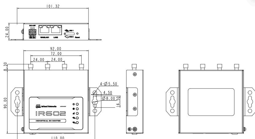
尺寸图
