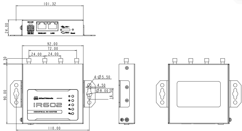
尺寸图
