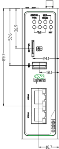
接口图
