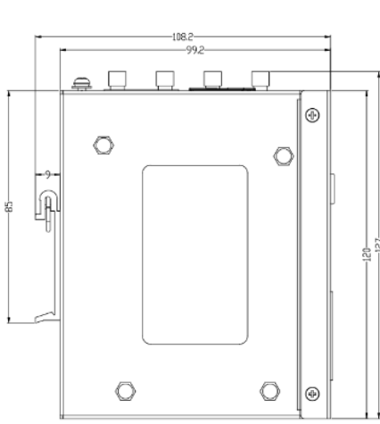
正视图
