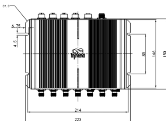
正视图
