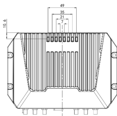
正视图
