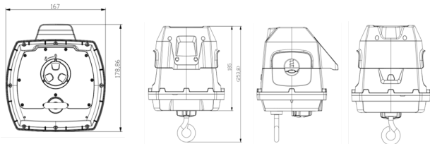
尺寸（长×宽×高）：179×167mm×185mm(含丝杠为254mm)
