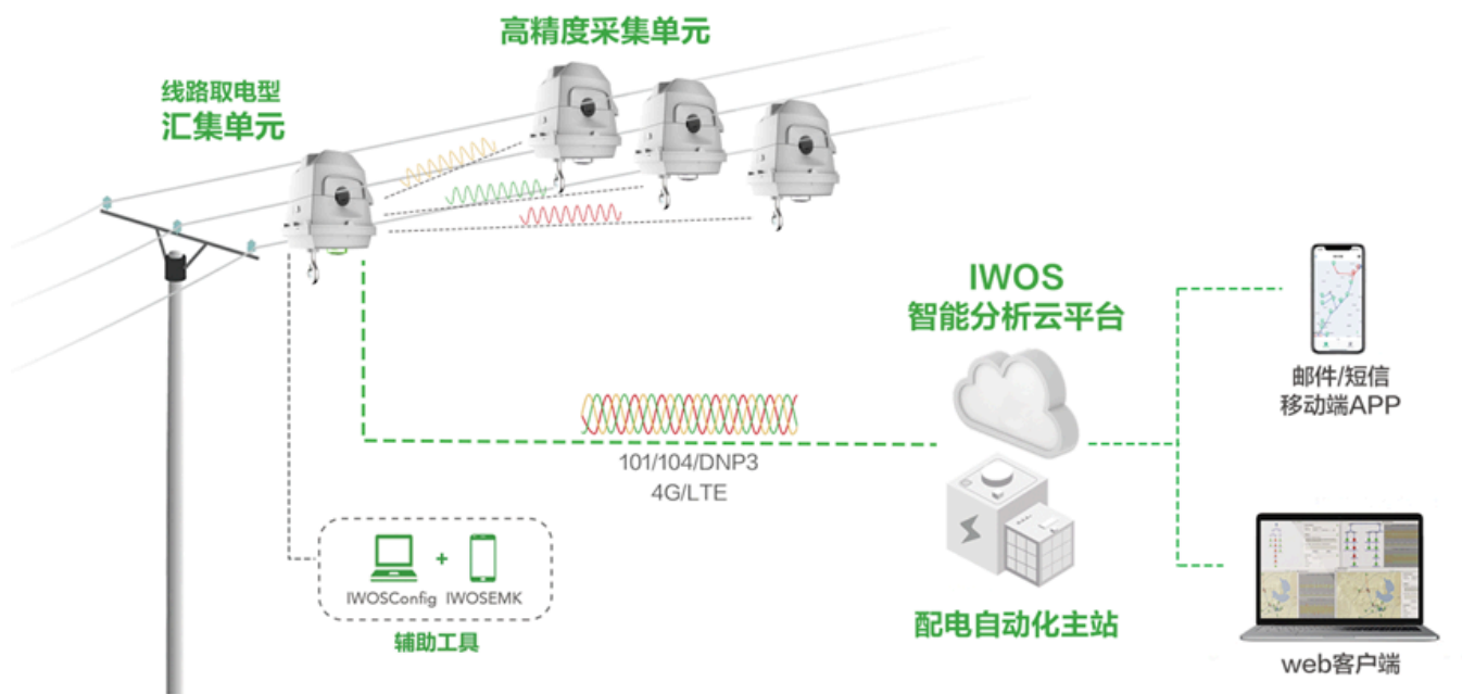
智能化配电网线路状态监测系统
