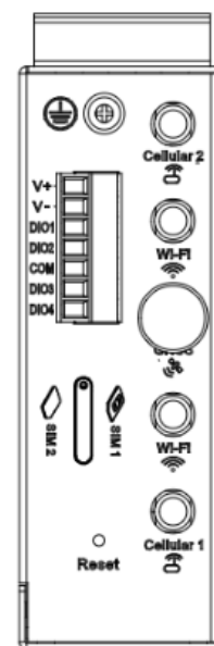
侧视图
